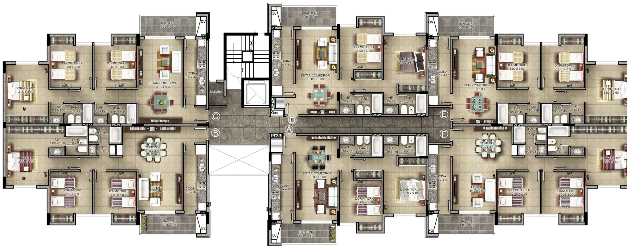
PLANTA TIPO 1º Y 2º PISO
